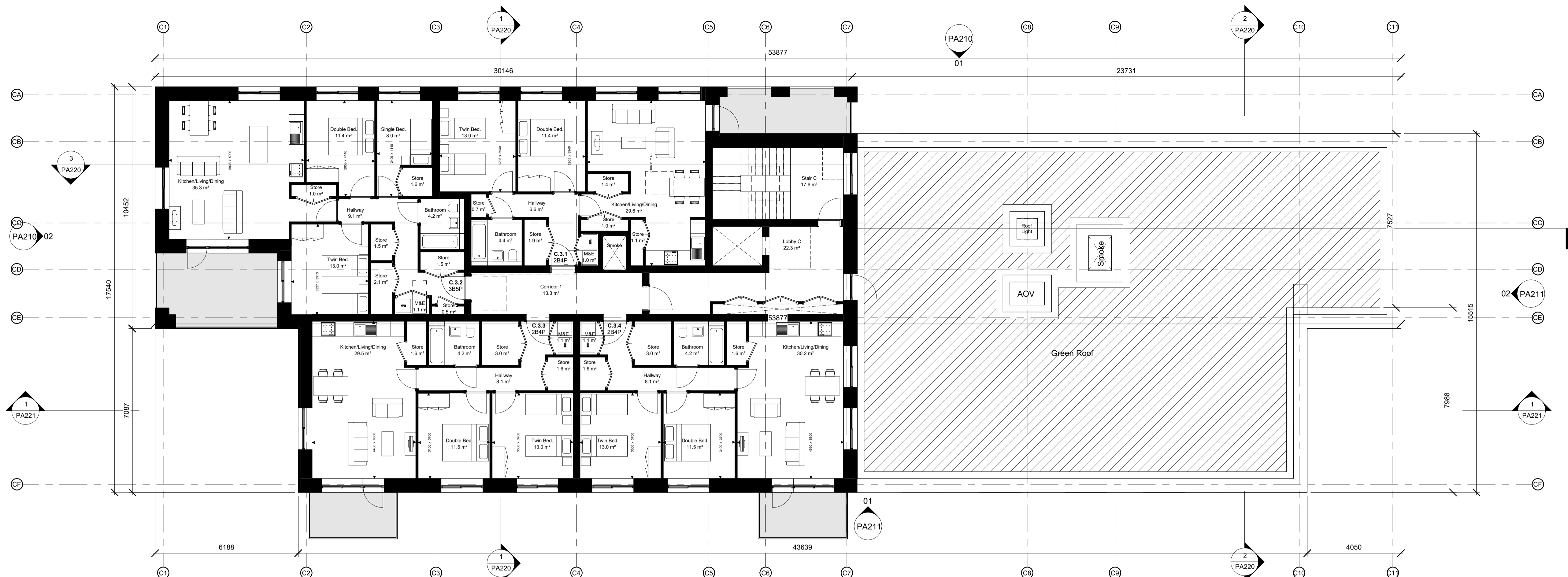
2 Apartment C_Level 03 1 : 100
