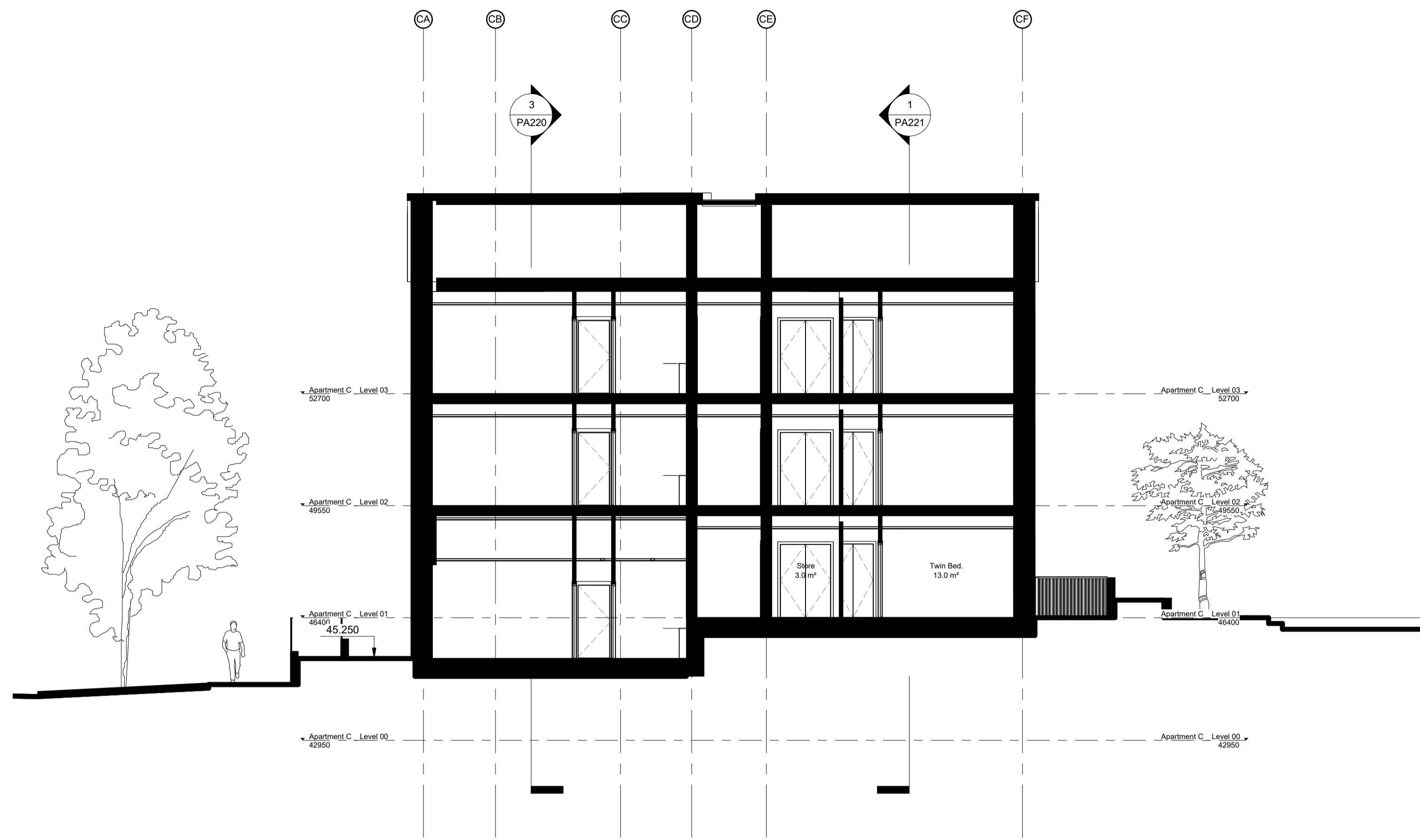
1 Block C - Section 1-1 1 : 100
