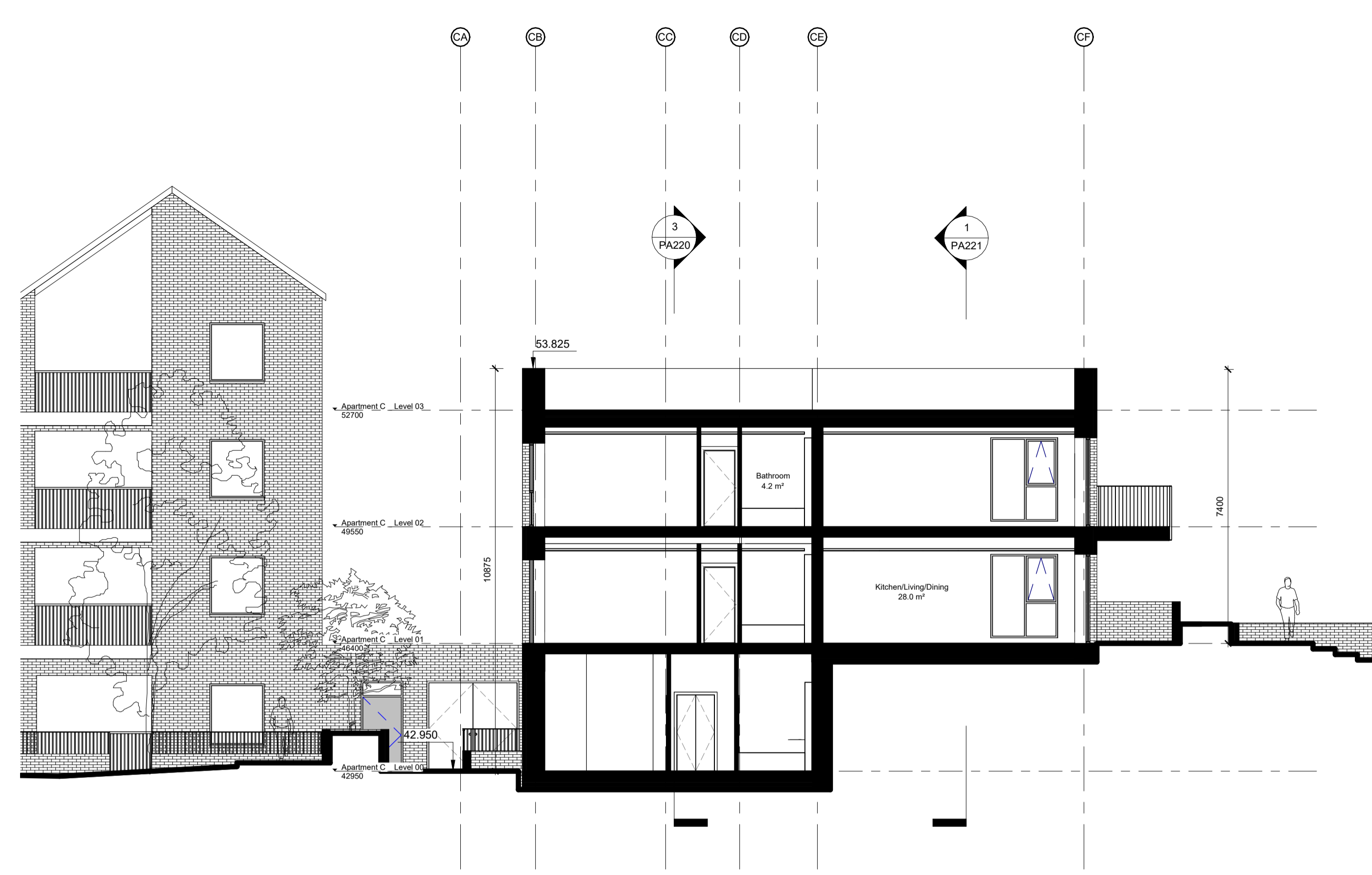
2 Block C - Section 2-2 1 : 100
