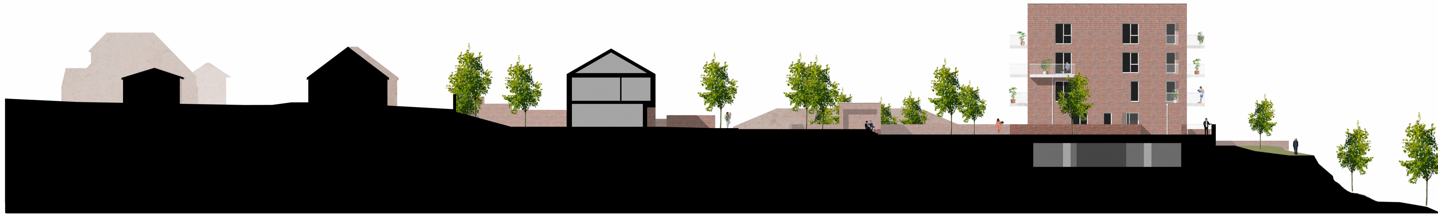
01 Site Section AA 1 : 250
