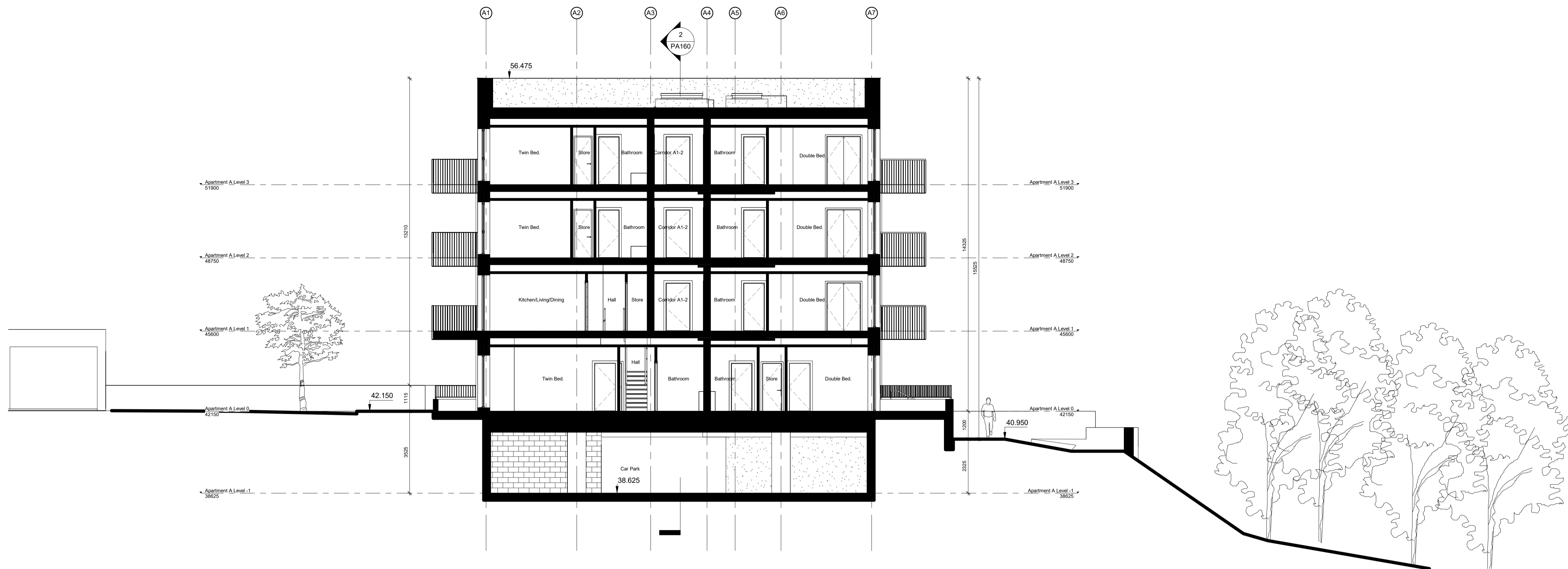
1 Block A - Section 1-1 1 : 100
