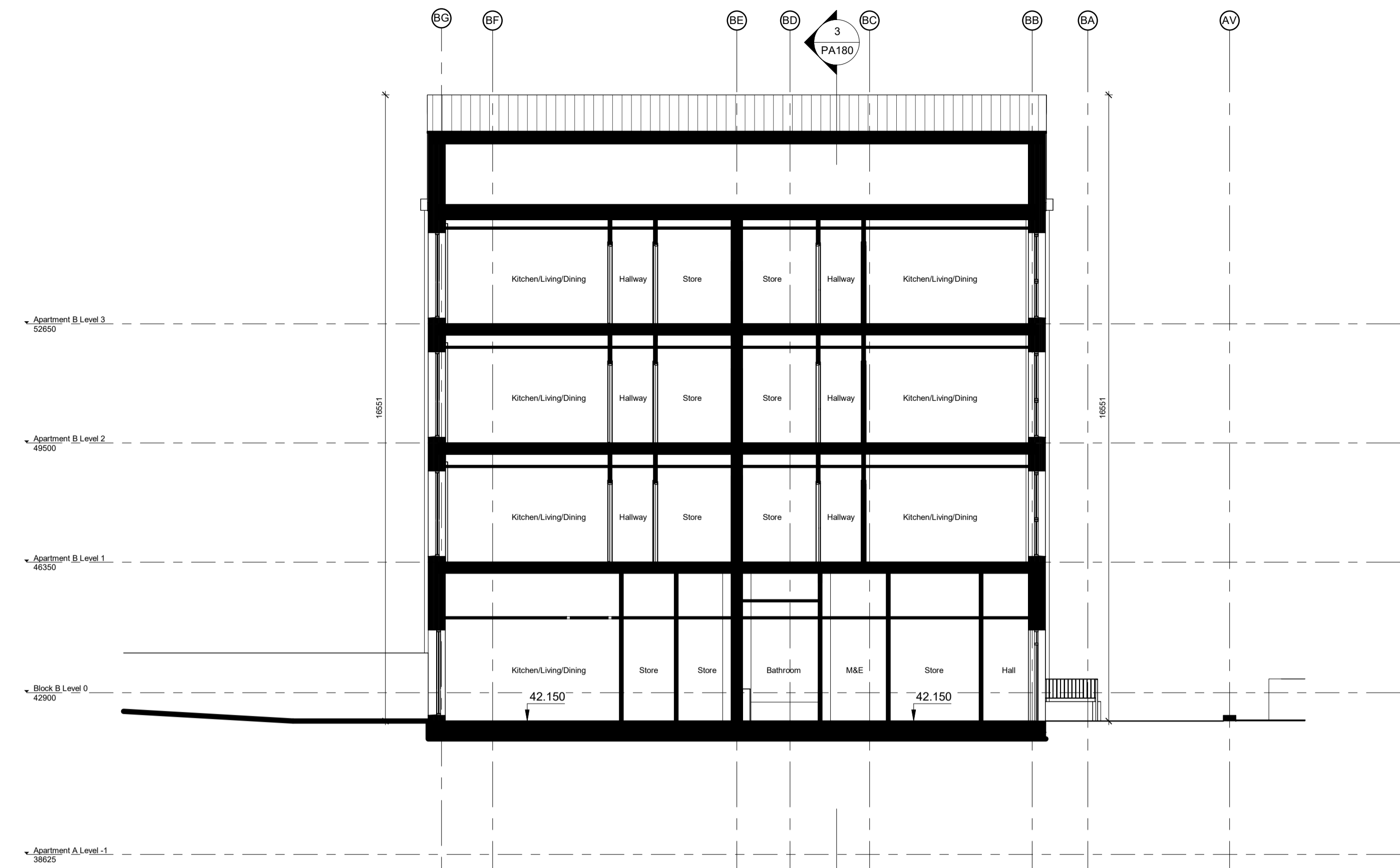
2 Block B - Section 2-2 1 : 100
