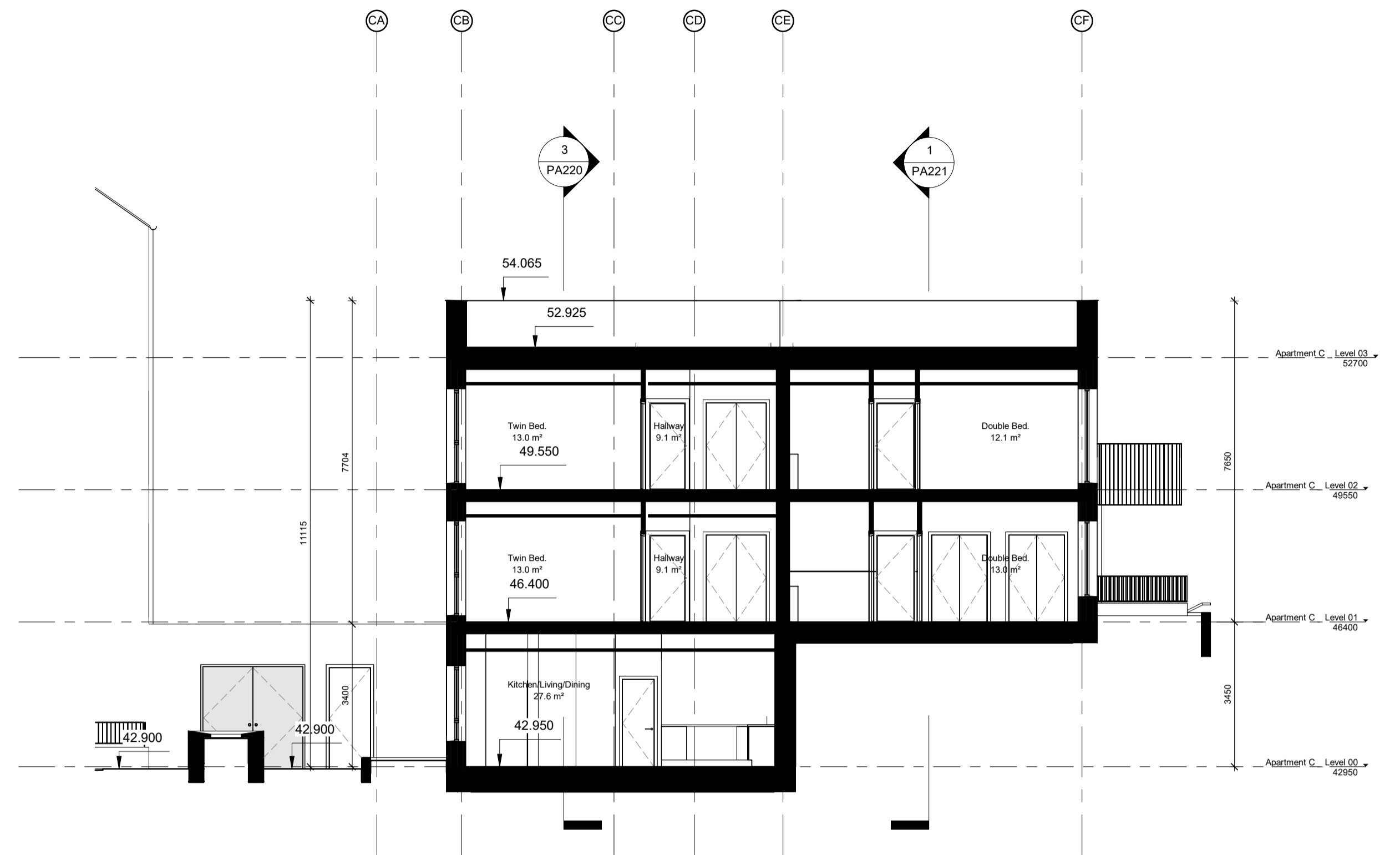
2 Block C - Section 2-2 1 : 100
