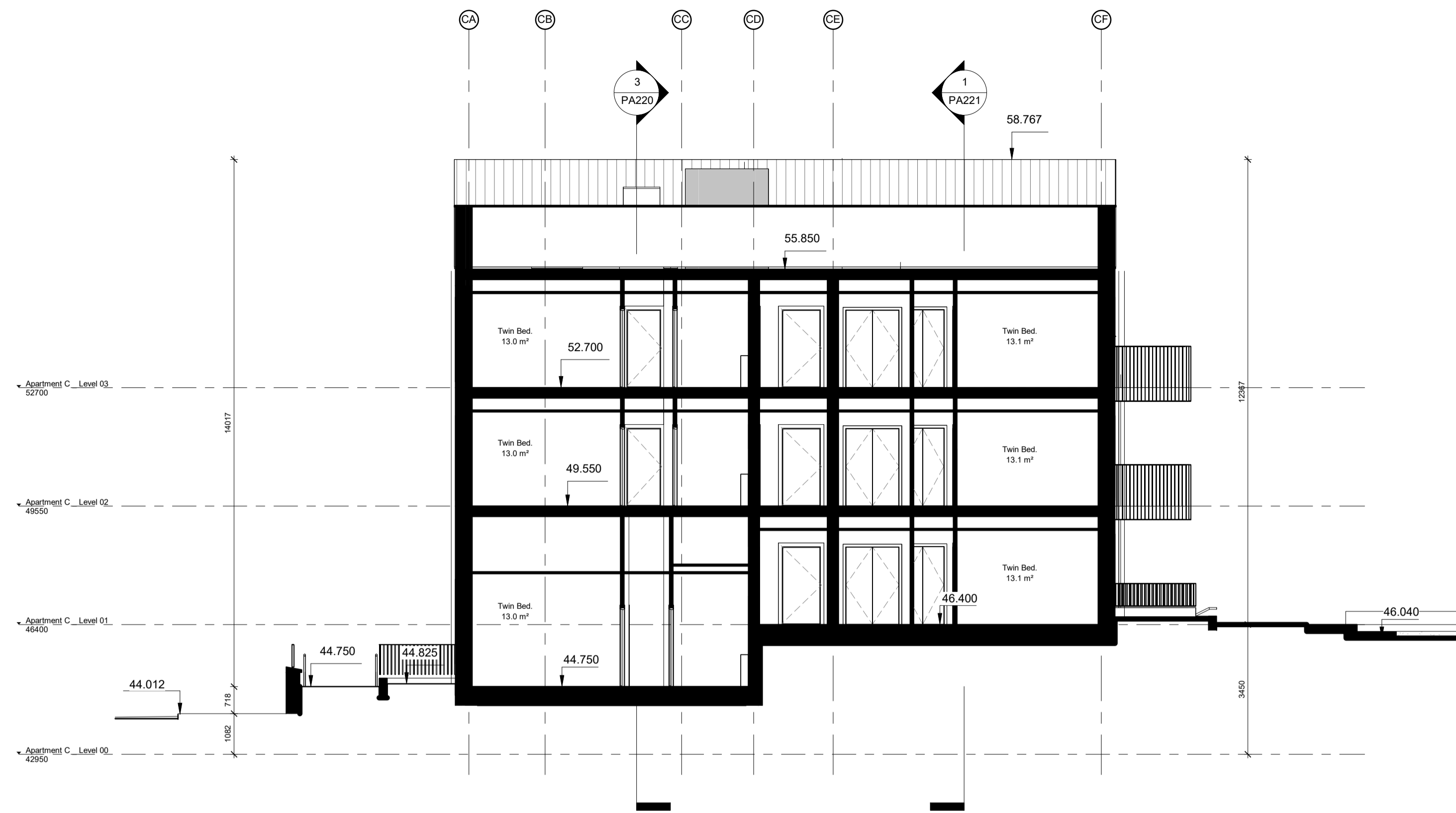
1 Block C - Section 1-1 1 : 100
