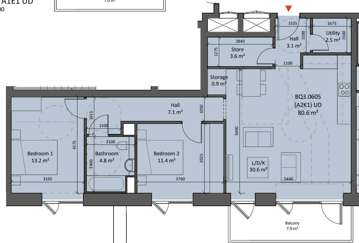
④ AT - A2K1 UD 1 : 100
