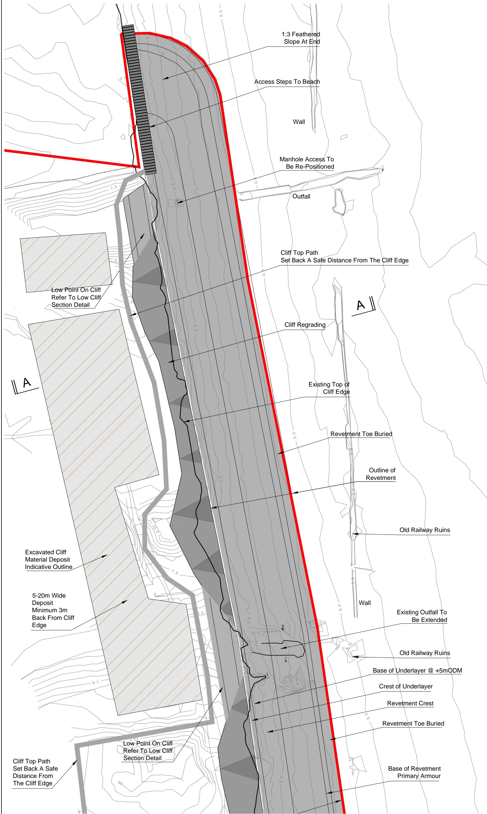
Site Layout Plan 1 SCALE : 1:500
