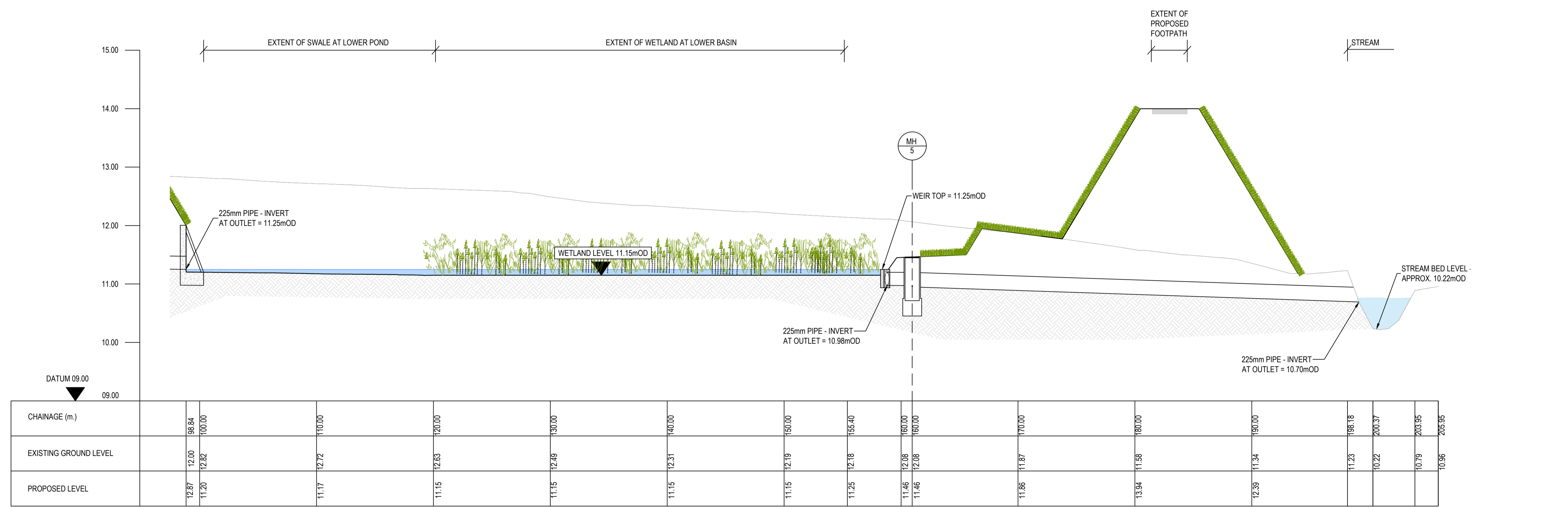
LONGSECTION A-A SCALE:H1:200, V1:40. DATUM: 9.00
