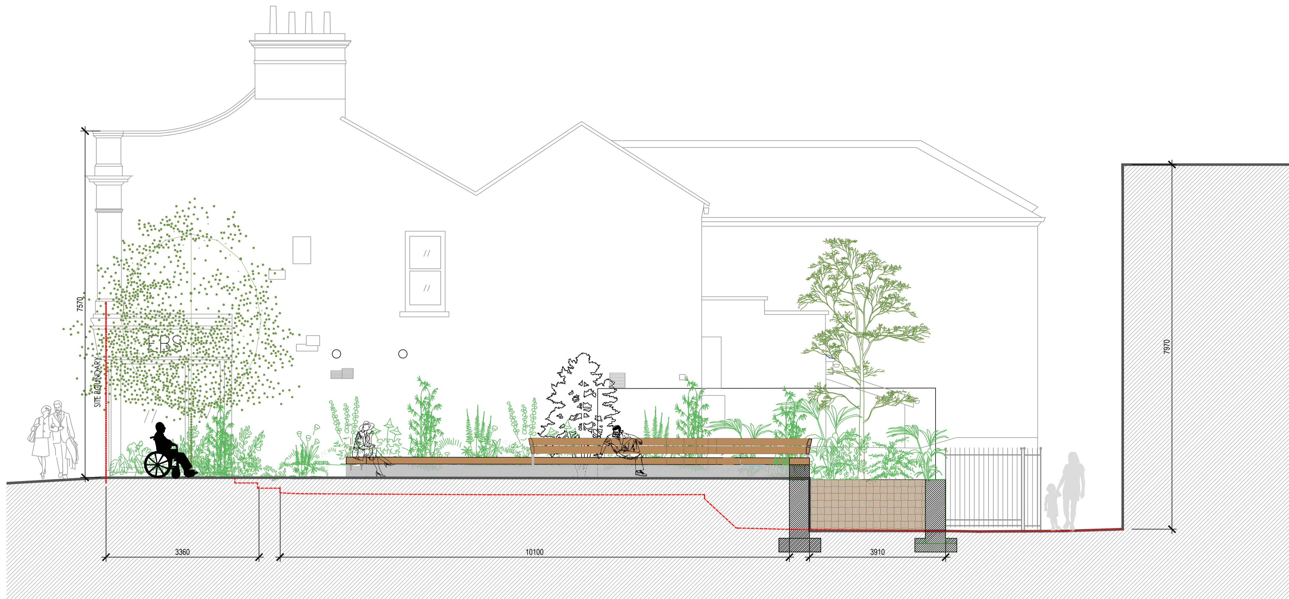
A SECTION A-A Scale: 1:50 @ A1
