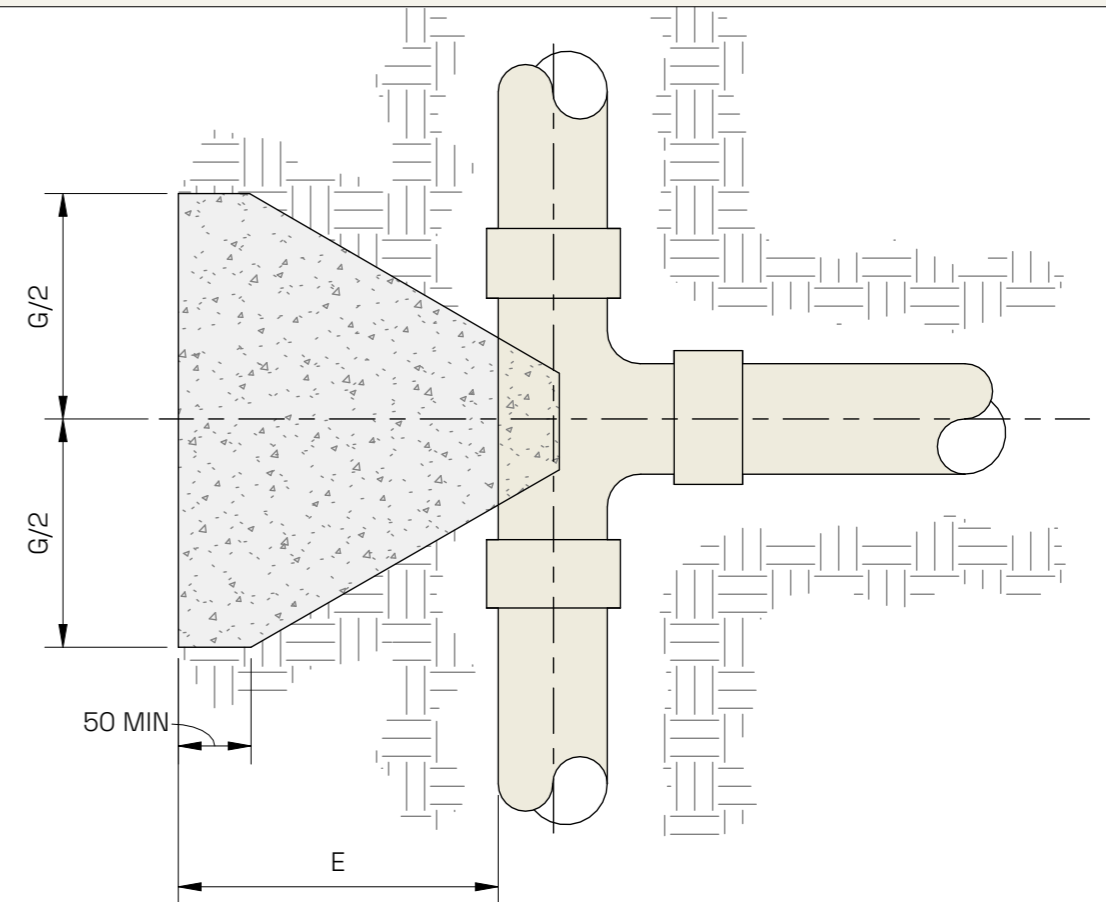
TEE
